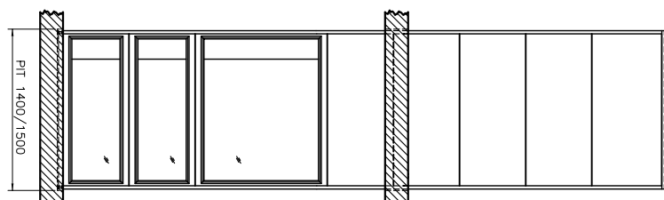
D-D 1:20
