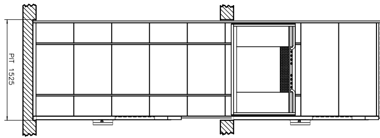
A-A 1:20
