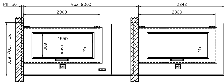
B-B 1:20
