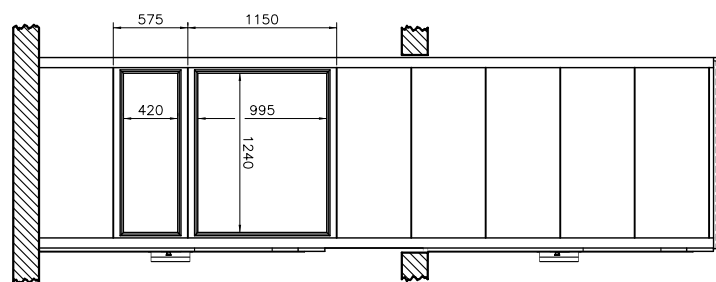
C-C 1:20
